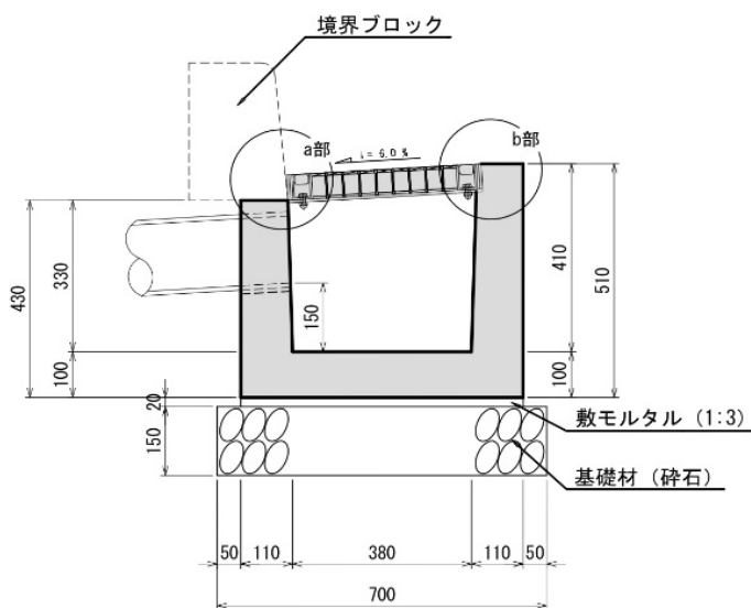
施工図（A-A断面）
