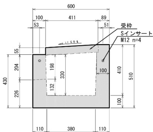
側面図（C-C矢視）
