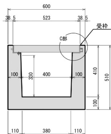
断面図（D-D）
