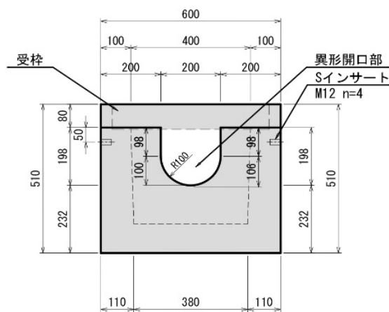
正面図（B-B矢視）
