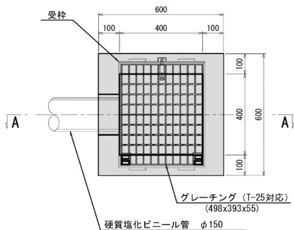
施工図（平面）
