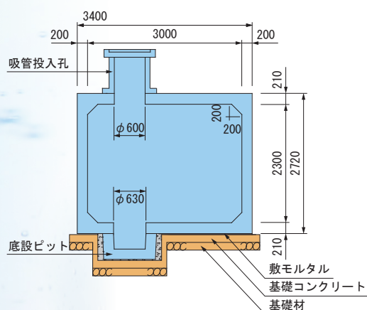
【断面図】
