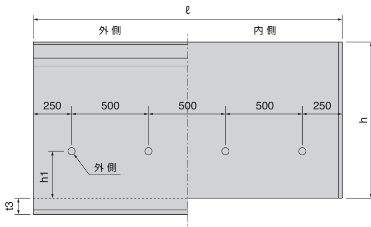
■側面図
