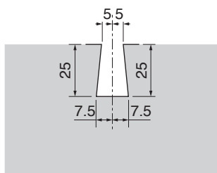
■目地詳細図
