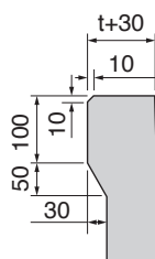
■側壁頂部詳細図
