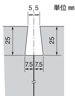
■目地詳細図
