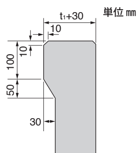
■側壁頂部詳細図
