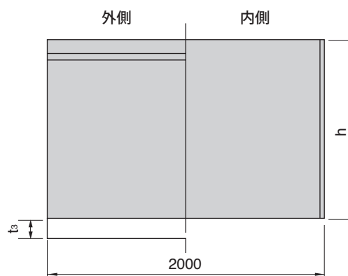
■側面図
