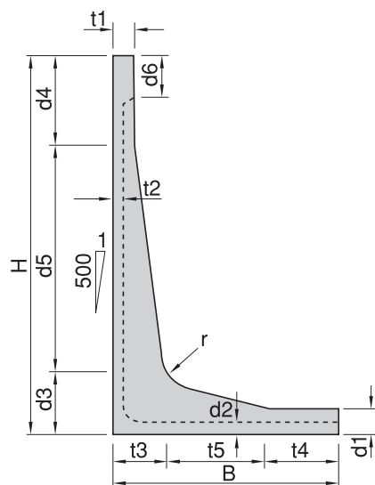
【側面図】
