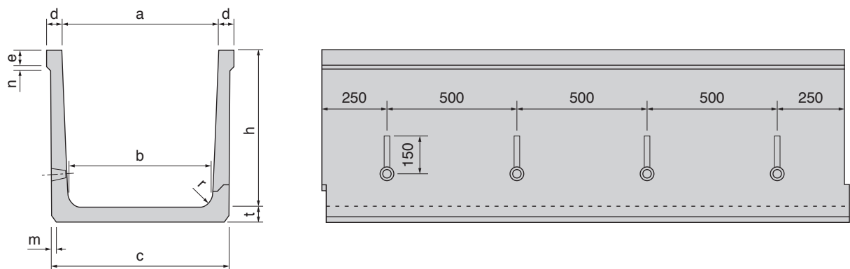
排水孔詳細
