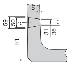
排水孔詳細
