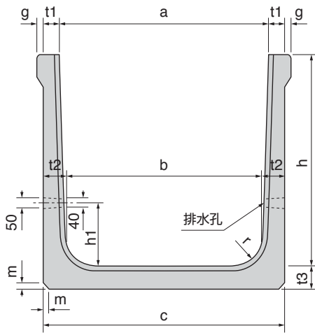
■断面図
