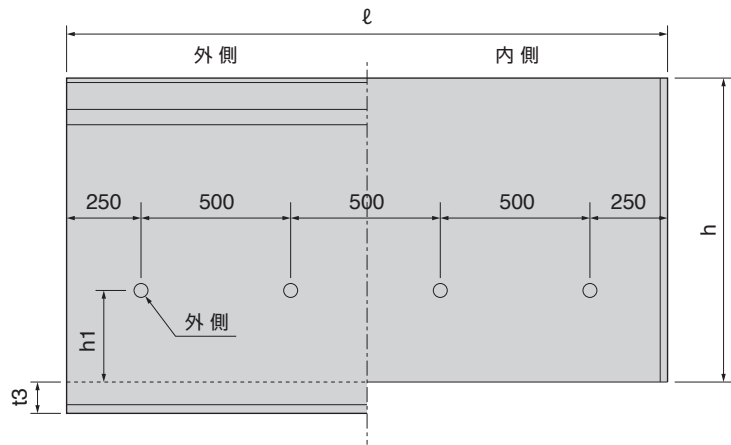
■側面図
