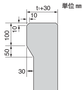
■側壁頂部詳細図
