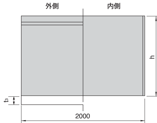
■側面図
