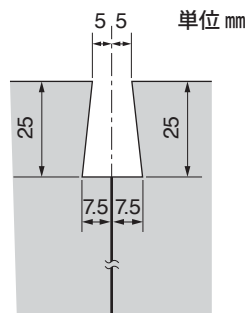
■目地詳細図
